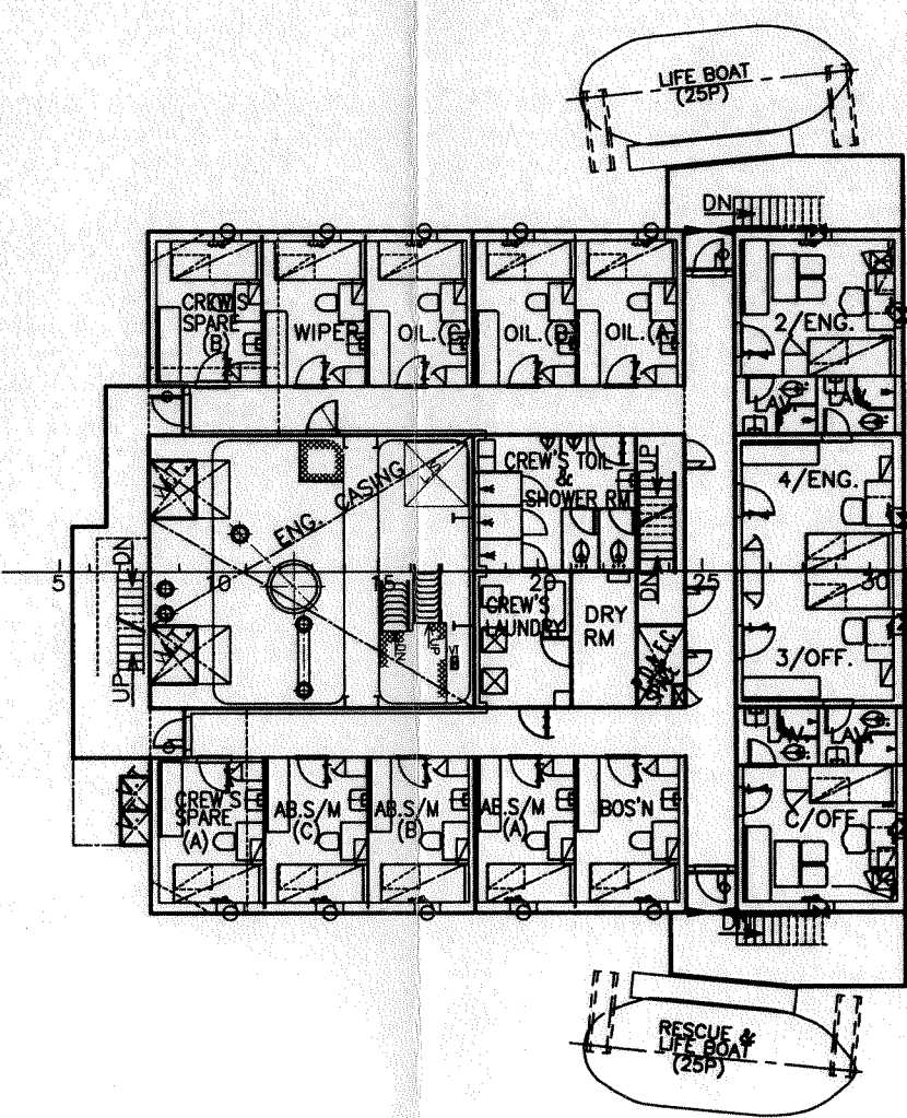
A-DECK
